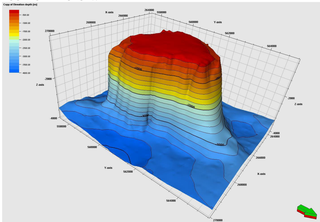
AFBEELDING 7 ZOUTKOEPEL ONSTWEDDE
