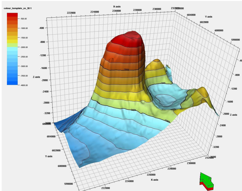
AFBEELDING 8 ZOUTKOEPEL PIETERBUREN
