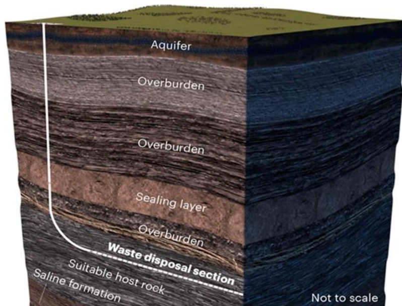
Figuur 4 Schema opslag kernafval via diep boorgat
