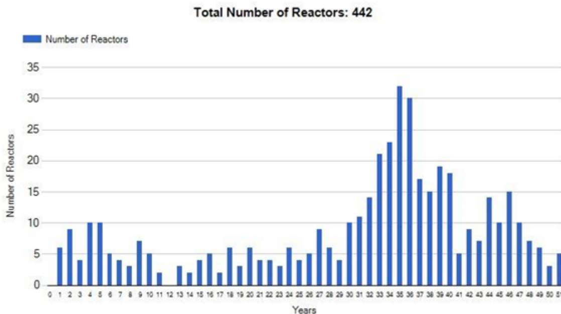
Figuur 1 Aantal jaren dat kerncentrales in bedrijf zijn
